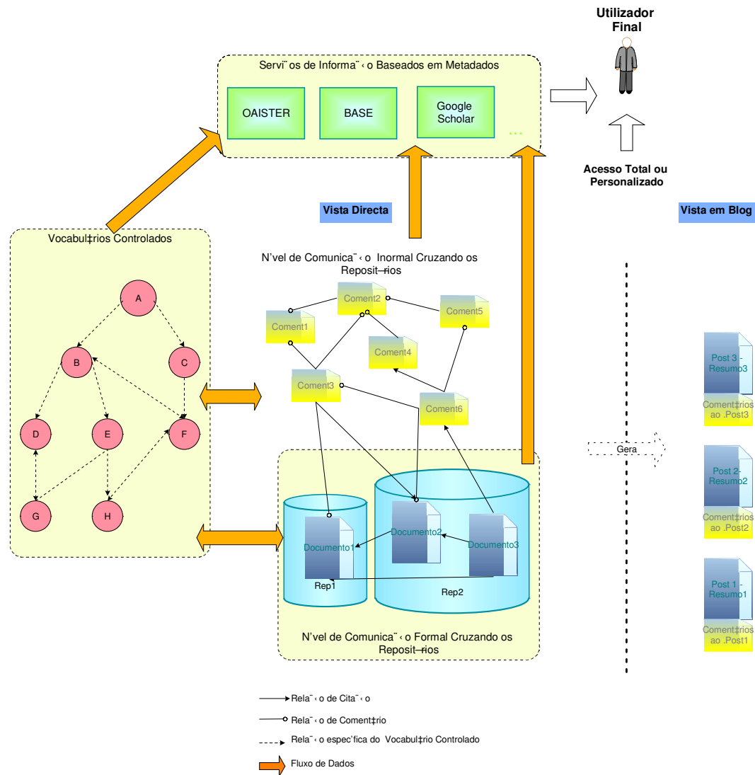
Figura 5 - Arquitectura final do novo serviço de comentários
